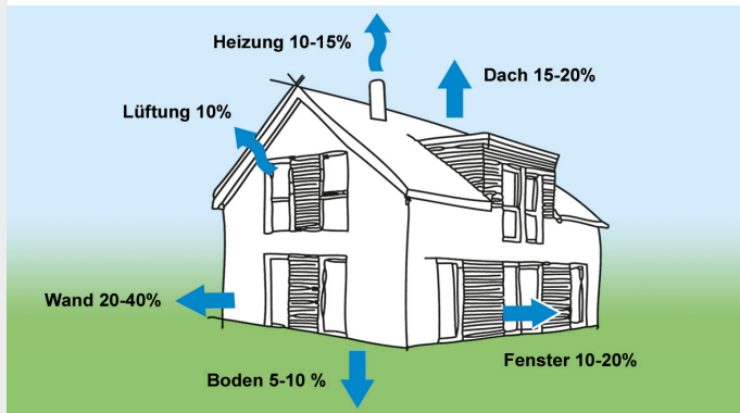
Wärmeverluste eines Altbaus
